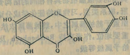
图 1 地梢瓜组中的黄酮醇
